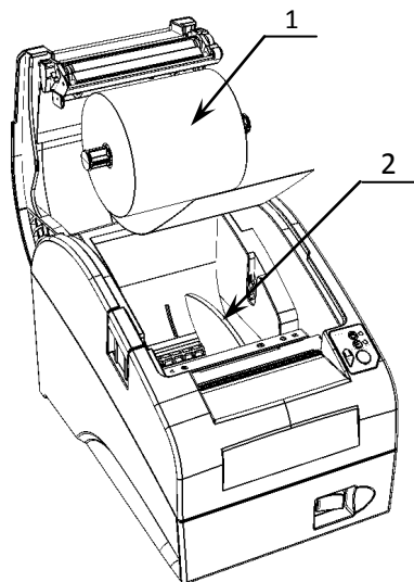
Рисунок 4. Заправка ЧЛ
